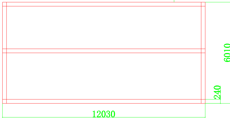
条形地基图
